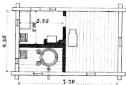
Wärterhaus mit Wasserstation. \frac{1}{250} .
