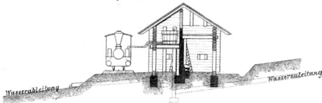
Fig. 22. Querschnitt. \frac{1}{250} .
