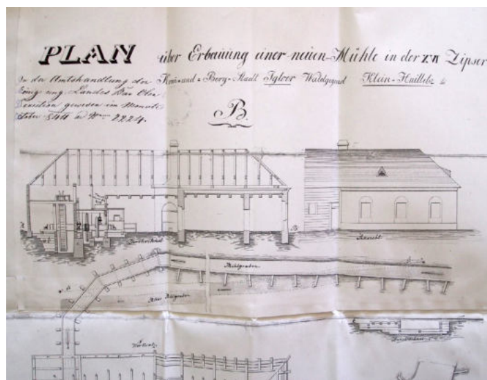
Výrez z plánu stavby nového mestského mlyna v hornej časti obce z roku 1844. (Mesarčíkov mlyn)
